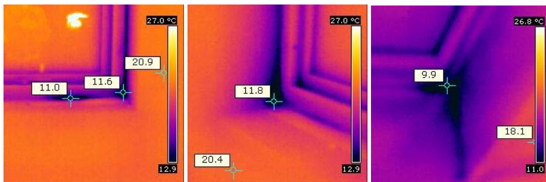
Fönster med typiska läckor i underkant och hörn. Kontrollerat under pågående byggnation
